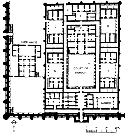
شكل (٢) مسقط أفقي لقصر الأخيضر عن: الحداد، المجلد، شكل (٥١).
