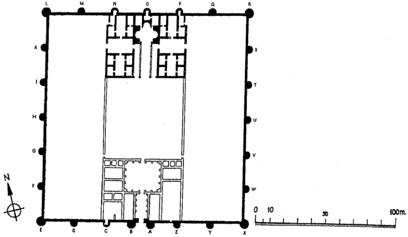
شكل (٥) مسقط أفقى لقصر الحير المشتى عن:
